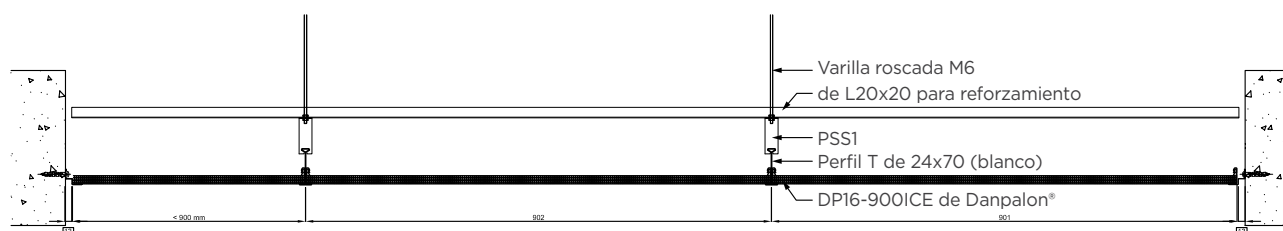
Corte A-A: En área de reforzamiento
